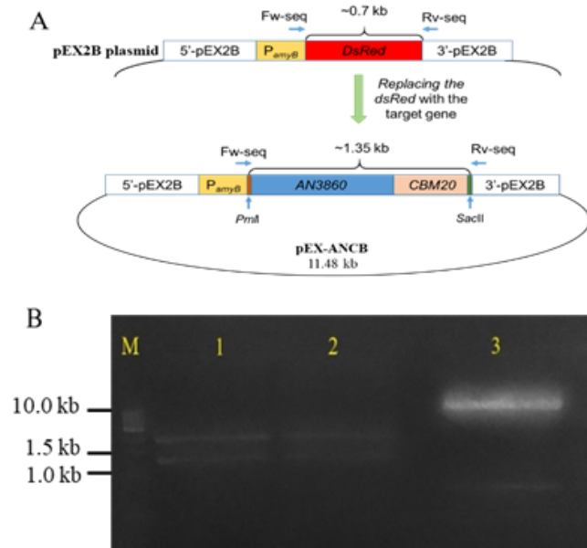
Fig. 1 AN3860-CBM20 vector construction
